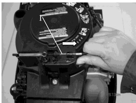
1. Käynnistyksenestovaijeri
