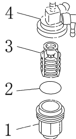
1. suodatinkuppi 2. O-rengas 3. suodatinelementti 4. suodattimen kansi
